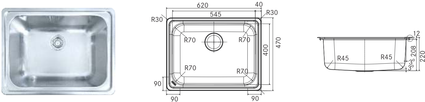
RSX 610-63 (24"x18")
