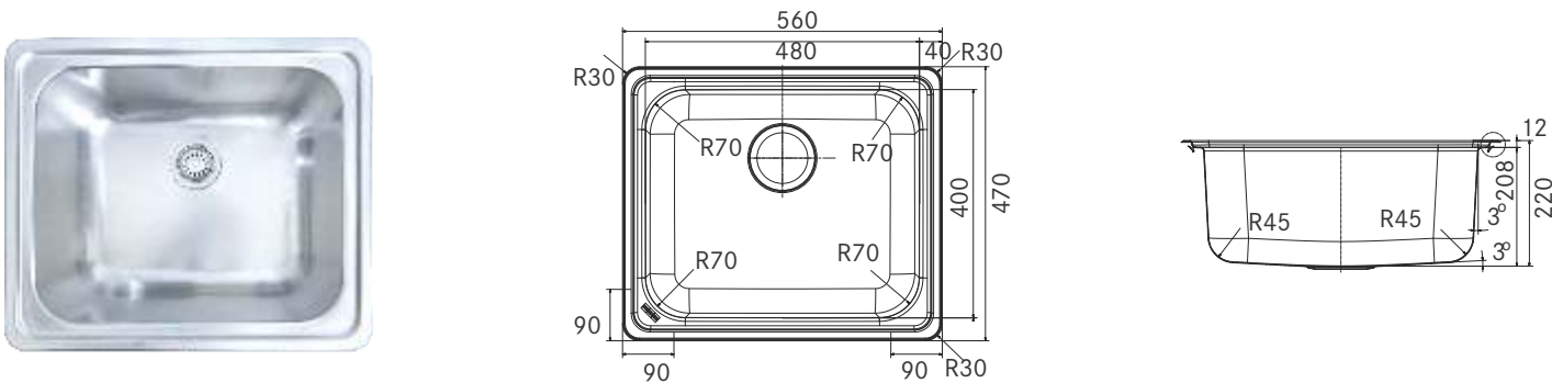
RSX 610-56 (22"x18")
